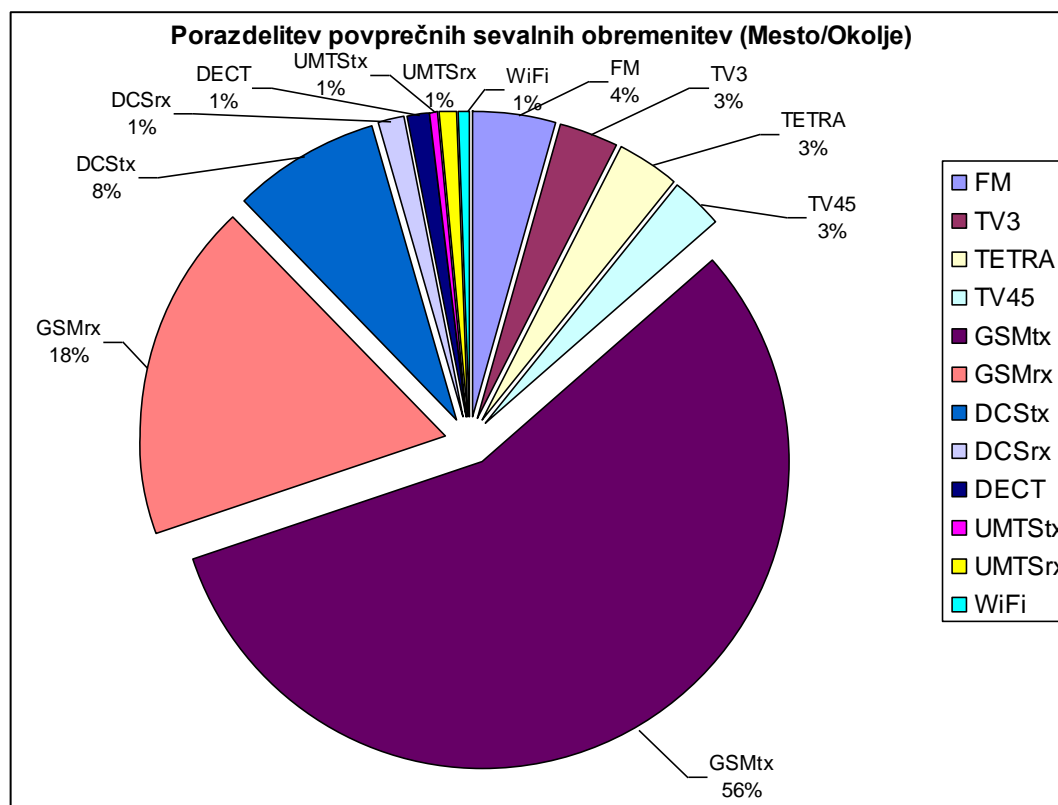
Slika 16: Posamezni prispevki iz različnih frekvenčnih področij k skupnim povprečnim sevalnim obremenitvam za mesto/okolje
