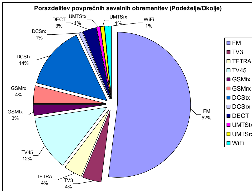
Slika 17: Posamezni prispevki iz različnih frekvenčnih področij k skupnim povprečnim sevalnim obremenitvam za podeželje/okolje.
