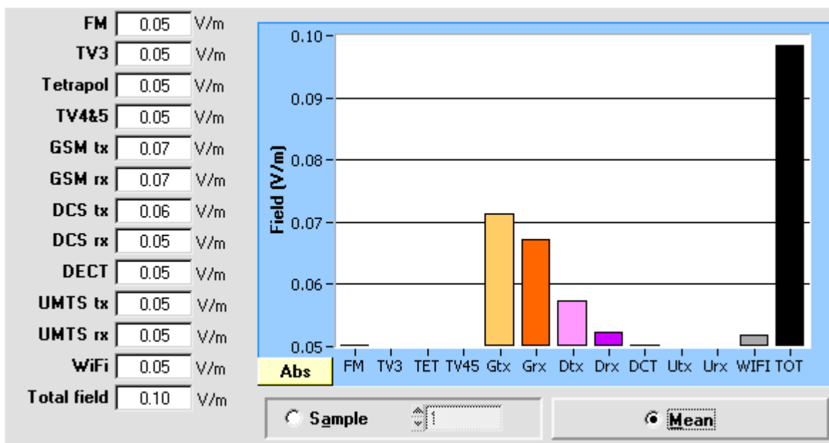
Slika 1: Povprečna vrednost izmerjenih vrednosti električne poljske jakosti po posameznih frekvenčnih področjih ter celotne vrednosti poljske jakosti zaradi vseh virov skupaj (TOT). FM-radijski oddajniki, TV3 in TV4&5-televizijski oddajniki, GSMtx-mobilni telefon v sistemu GSM 900; GSMrx-bazna postaja v sistemu GSM 900; DCS tx-mobilni telefon v sistemu DCS; UMTStx-mobilni telefon v sistemu; UMTSrx-bazna postaja v sistemu UMTS
