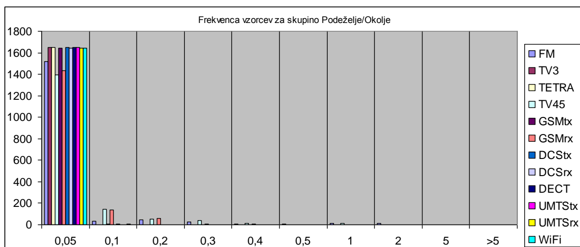
Slika 22: Histogram vzorcev za skupino Podeželje/Okolje
