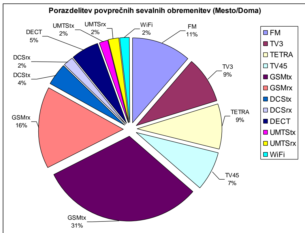
Slika 13: Posamezni prispevki iz različnih frekvenčnih področij k skupnim povprečnim sevalnim obremenitvam za Mesto-Doma.
