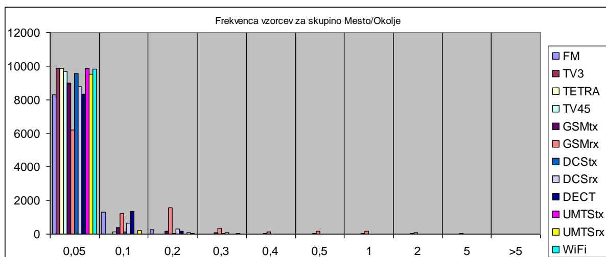
Slika 21: Histogram vzorcev za skupino Mesto/Okolje
