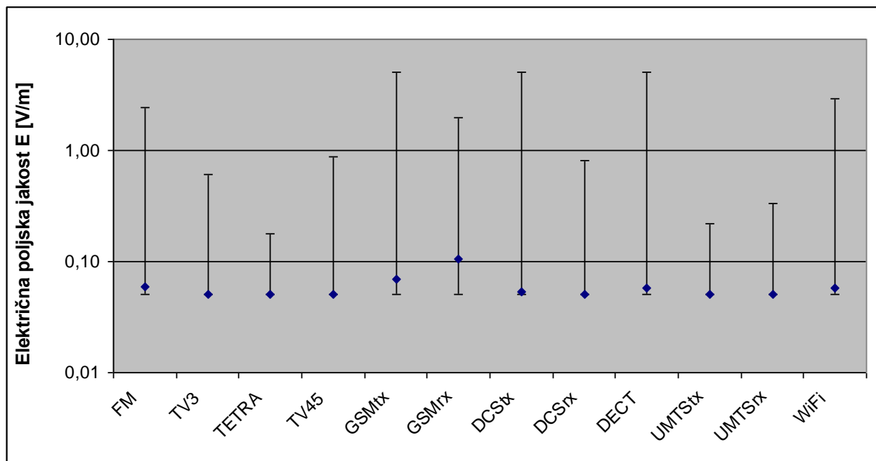
Slika 11: Povprečne, minimalne in maksimalne vrednosti za vse skupine združene skupaj.
