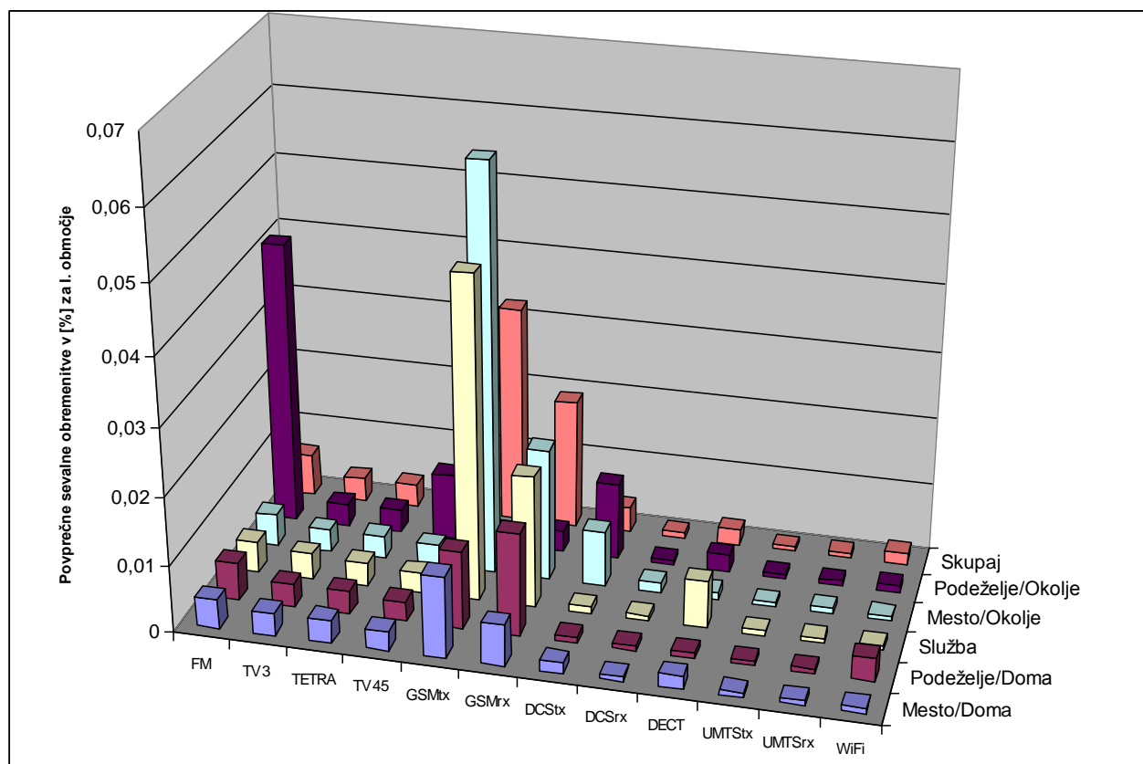
Slika 4: Maksimalne sevalne obremenitve za vseh pet področij izpostavljenosti. Vrednosti so v odstotkih mejne vrednosti glede na uredbo o elektromagnetnem sevanju za I. področje.
