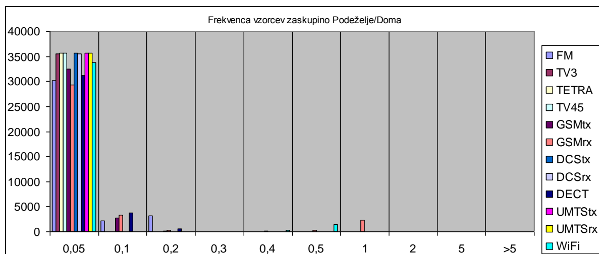
Slika 19: Histogram vzorcev za skupino Podeželje/Doma
